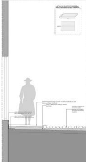
PARTICOLARI PAVIMENTAZIONI
